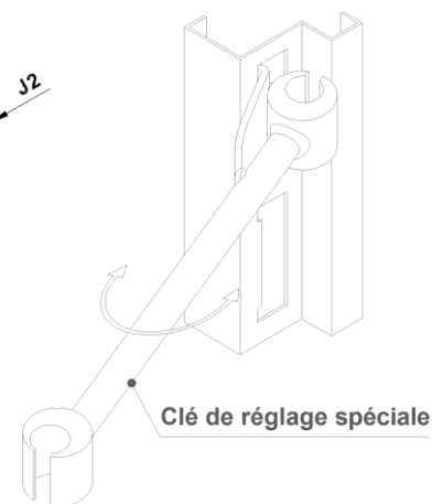
Côté paumelles universelle Et empennage
