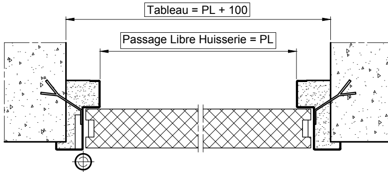
RESERVATION MACONNERIE SANS FEUILLURE
