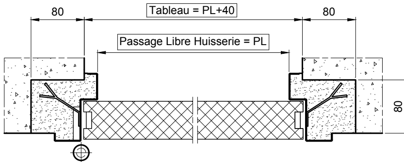
RESERVATION MACONNERIE AVEC FEUILLURE
