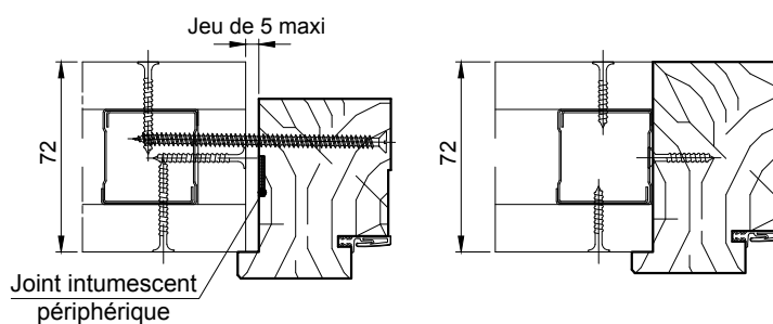
Schéma n°1 Pose après coup
