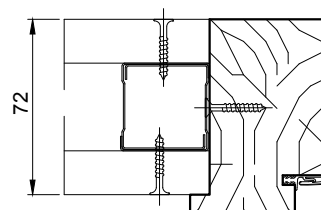
Schéma n°2 Pose à l'avancement
